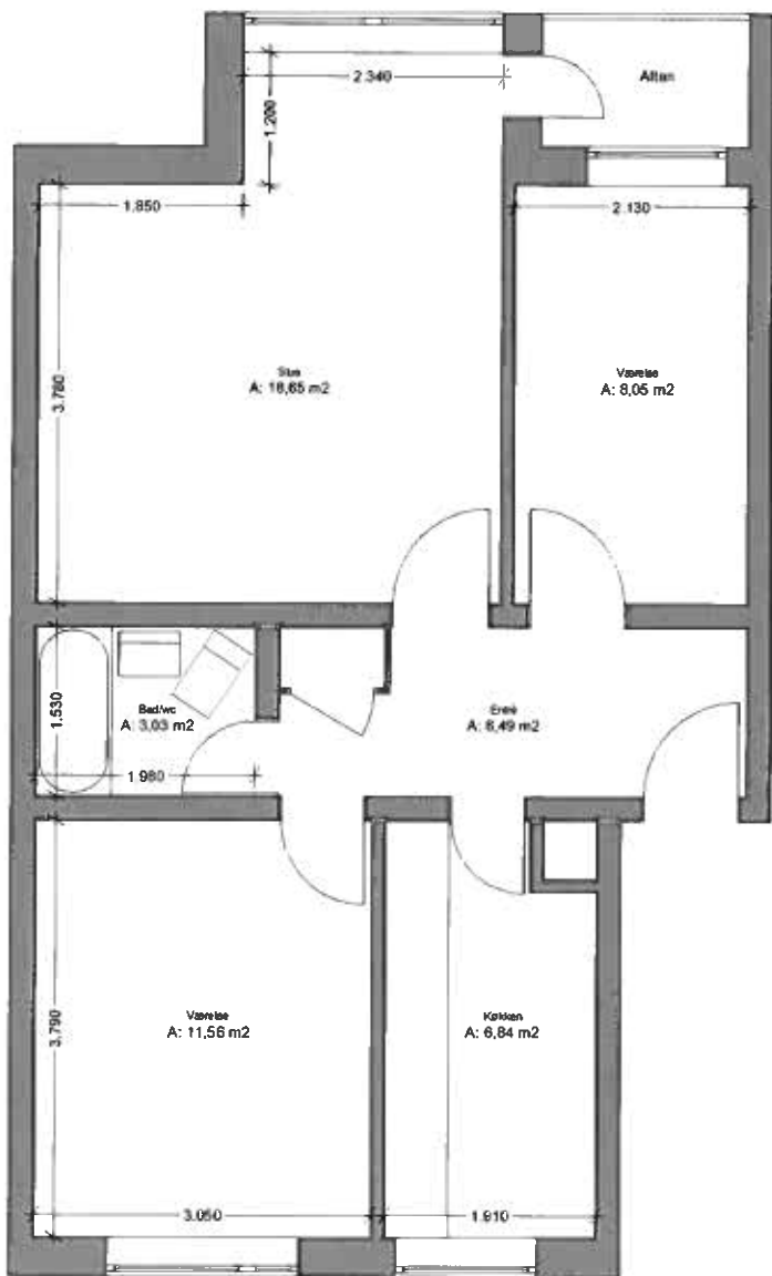
Stue-, 1. -, 2. -, & 3. salsplan
