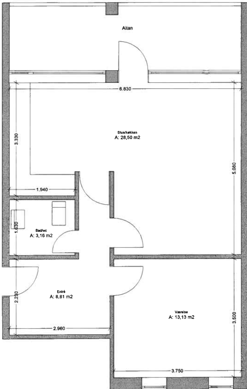
3. salsplan
